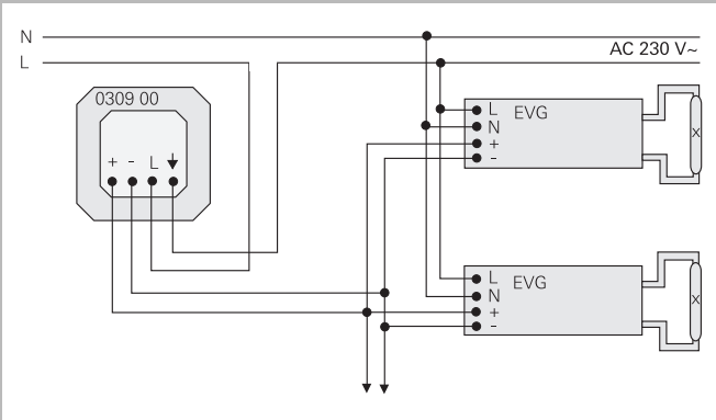
Подключение электронного потенциометра с функцией клавишного выключателя на EVG
