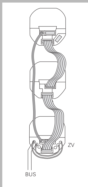
Подключение домофона при соединении „Шлейф“
