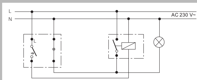
Кнопка (выключатель с нормально-разомкнутым сигнальным контактом)
