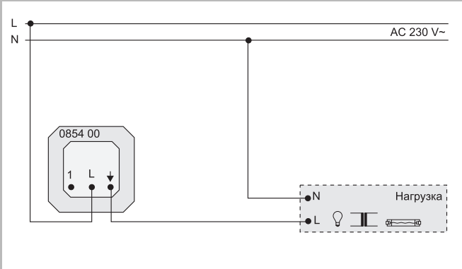
Подключение вставки выключателя TriacSystem 2000
