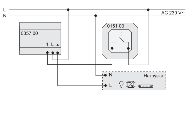
Подключение светорегулятора Tronic REG
