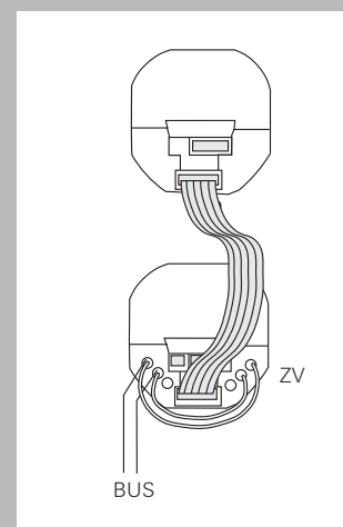
Подключение домофона при соединении „Последовательная цепь“
