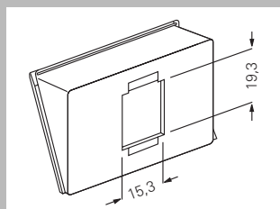
Вставка к модульному разъему Jack/Western Technik, AMP/Radiall, 1-секционн. 0052 00
