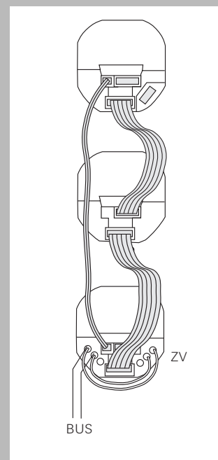
Подключение домофона при соединении „Последовательная цепь“
