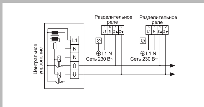
Параллельное включение разделительного реле 0386 00
