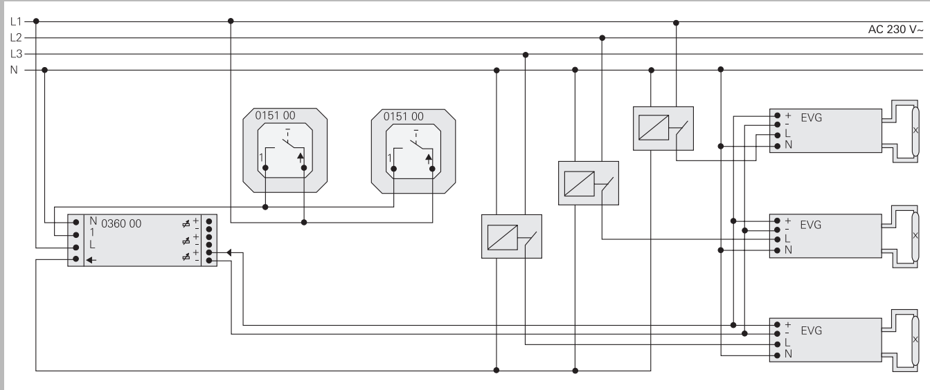
Подключение встраиваемого модуля управления с выходом 1–10 В на 3 фазы
