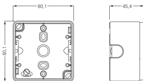
Корпуса для открытой электропроводки
