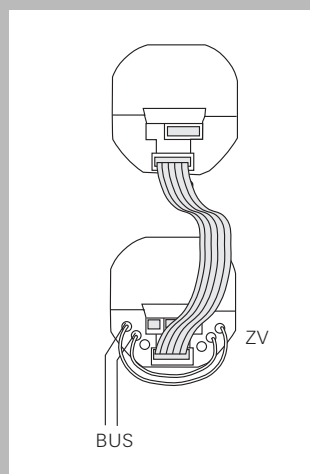
Подключение домофона при соединении „Шлейф“
