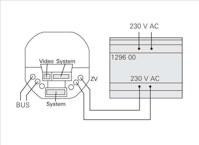
Соединения с клеммной колодкой шины
