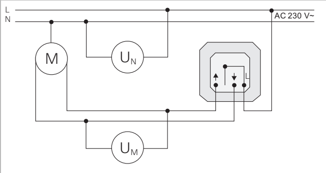
Измерение моментального напряжения сети U_N и напряжения электромотора U_M
