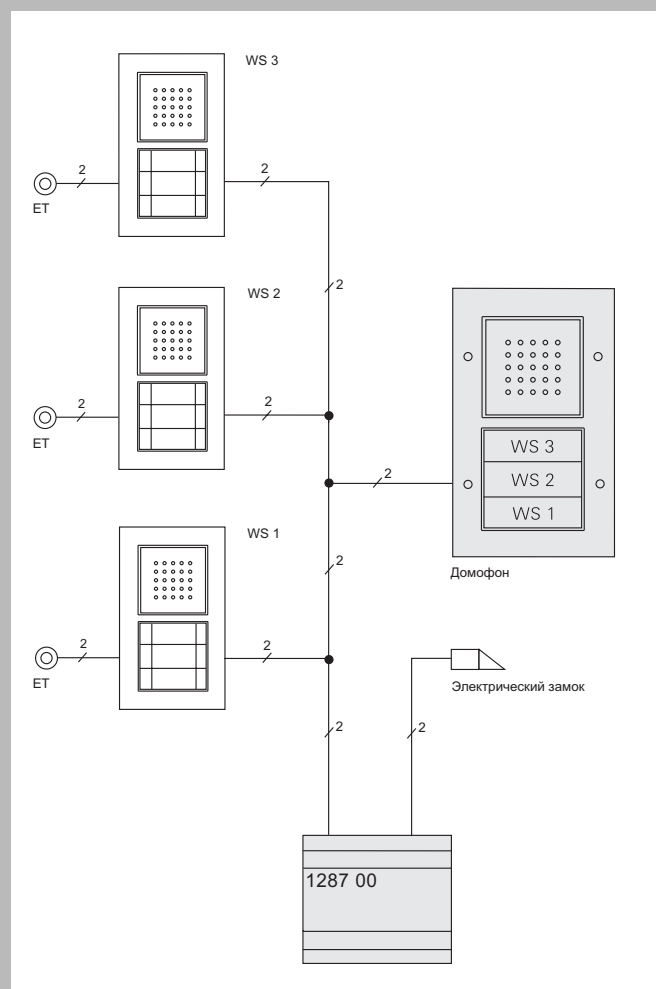
Способ соединения „Шлейф“
