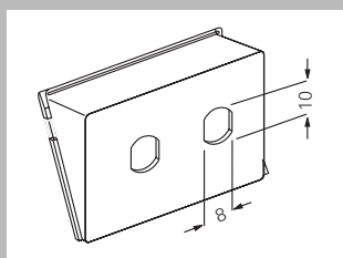
Вставка к волоконно-оптическому кабелю ST 2.5 мм 0732 00
