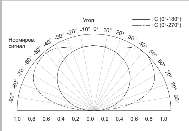
Характеристика излучения в полярных координатах
