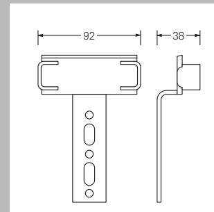
Габариты сборной опоры короба 0828 00
