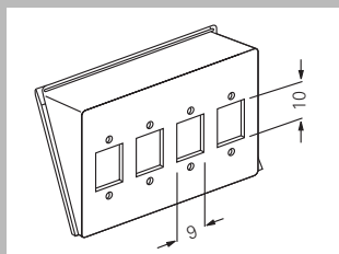
Вставка к симплексному разъему для волоконно-оптического кабеля SC, 4-секционн. 0090 00
