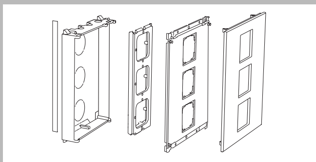
Унифицированный модуль для установки трех вставок для скрытой электропроводки серии System 55 в модульные функциональные стойки.
