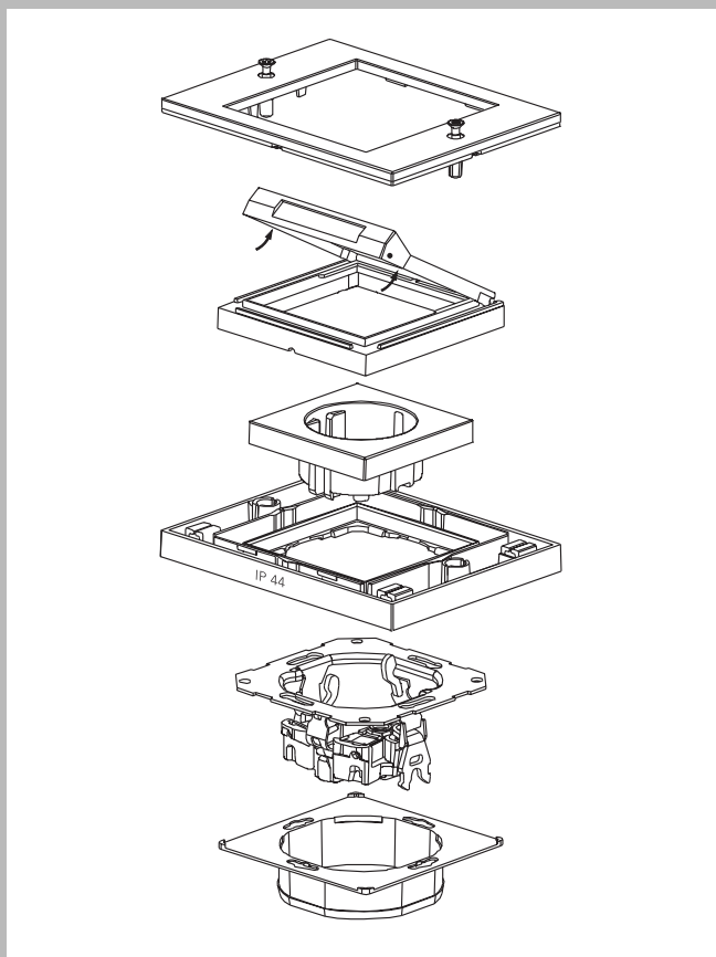
Установка вставок для скрытой проводки серии System 55
