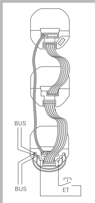
Подключение квартирной станции при соединении „Последовательная цепь“
