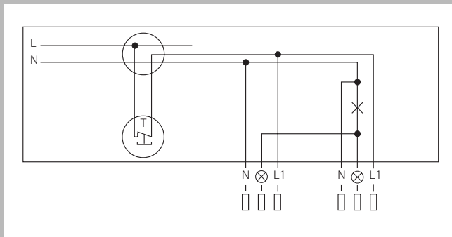
Включение нескольких контрольных устройств (параллельное включение)
