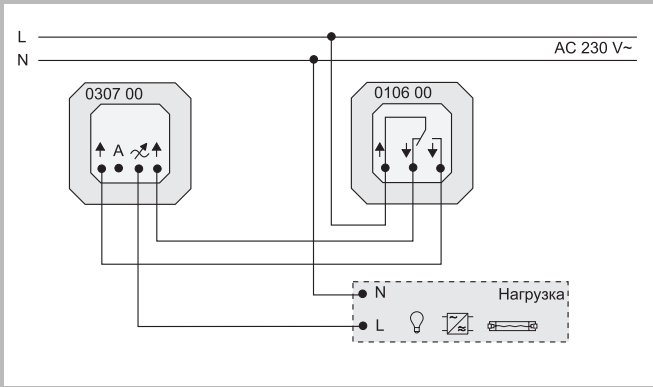
Включение с двух разных мест
