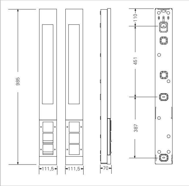
Габариты панели со световым элементом, выключателем и двумя розетками с заземляющими контактами. Габариты панели с тремя свободными гнездами.
