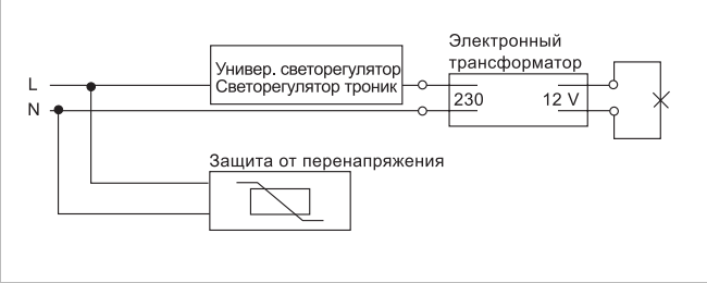
Режим работы со светорегулятором и с защитой от перенапряжения
