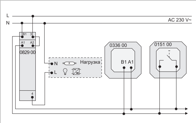
Подключение 3-проводного выключателя (переключаемый нулевой провод)
