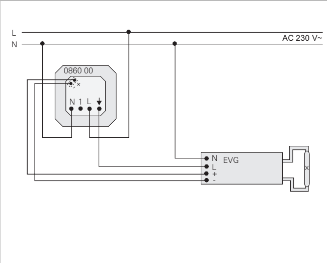
Вставка устройства управления 1–10 В
