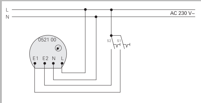
Подключение клавишных выключателей (выключатели с нормально-разомкнутым контактом S1, S2)
