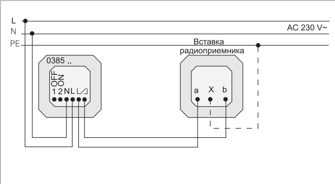
Подключение таймера к беспотенциальному параллельному входу вставки радиоприемника
