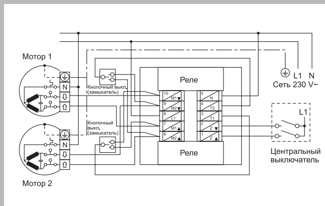
Схема соединения разделительного реле 0387 00
