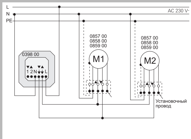
Параллельное включение моторов
