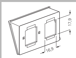
Вставка к модульному разъему Jack/Western Technik, Lucent (AT + T), 2-секционн. 0058 00
