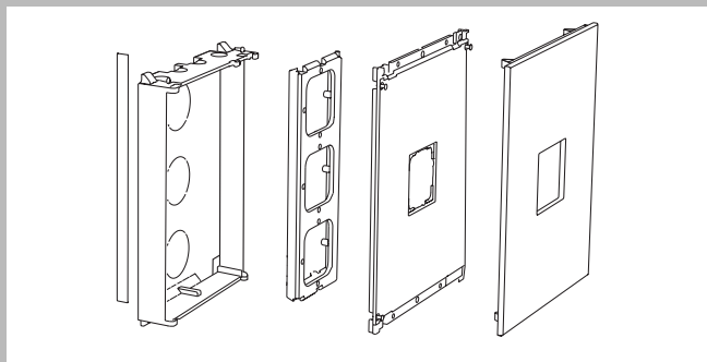
Унифицированный модуль для установки вставки для скрытой электропроводки серии System 55 в модульные функциональные стойки.
