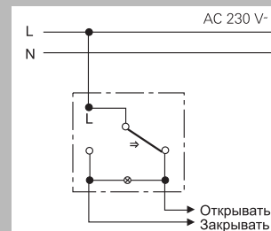
Кнопка (выключатель с переключающим контактом)
