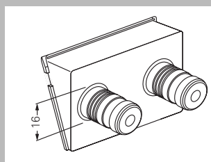
Вставка с встроенным разъемом для подключения акустических систем класса High-End WBT (+/-) 0091 00
