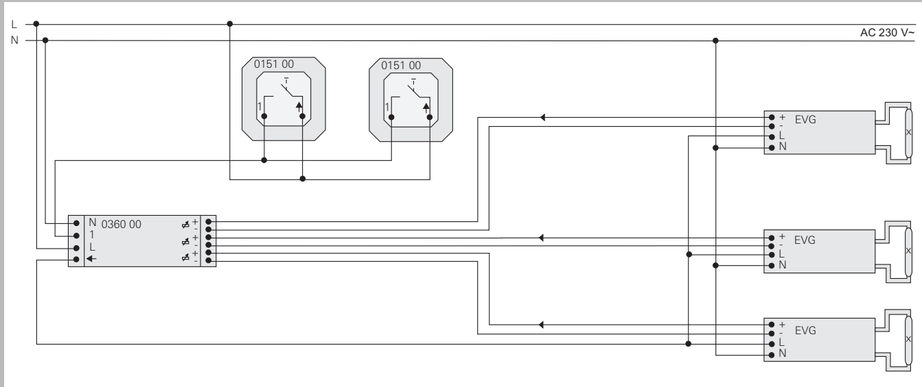
Подключение встраиваемого модуля управления с выходом 1–10 В
