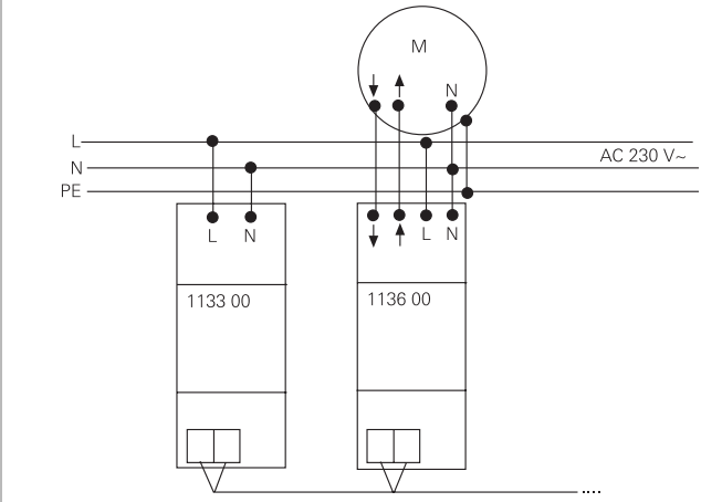
Подключение исполнительного радиоустройства управления жалюзи REG
