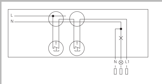
Включение с двух разных мест имеющийся выключатель может заменяться кнопочным выключателем „Т“ (с размыкающим контактом).
