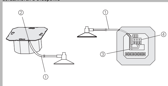
Сеть с открытой электропроводкой, вариант 1 (кнопочный выключатель управления с преобразователем сигналов датчика)
