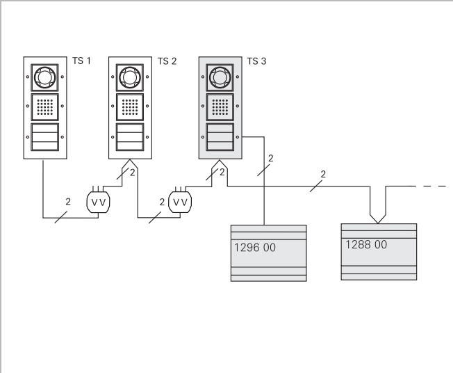
Подключение нескольких видеокамер
