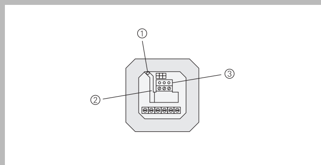
Подключение датчика для скрытой проводки
