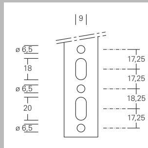
Расстояния между отверстиями сборных опор короба 0827 00, 0828 00
