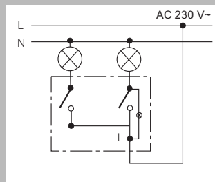
Двухклавишный выкл.
