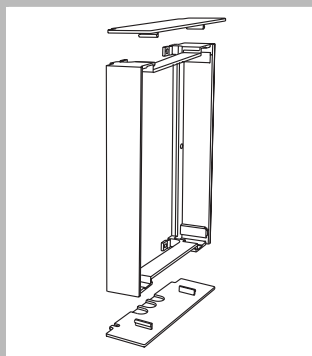
Монтажная рамка открытой проводки для установки модулей, 1251 04
