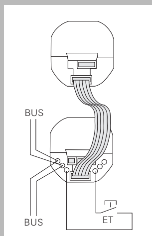
Подключение квартирной станции при соединении „Последовательная цепь“
