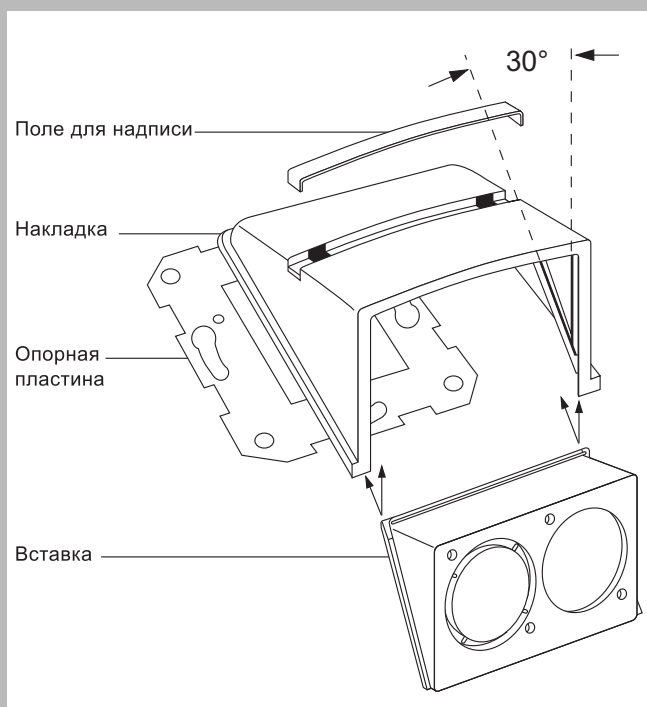
Накладка к розеткам для подключения средств связи и обмена данными
