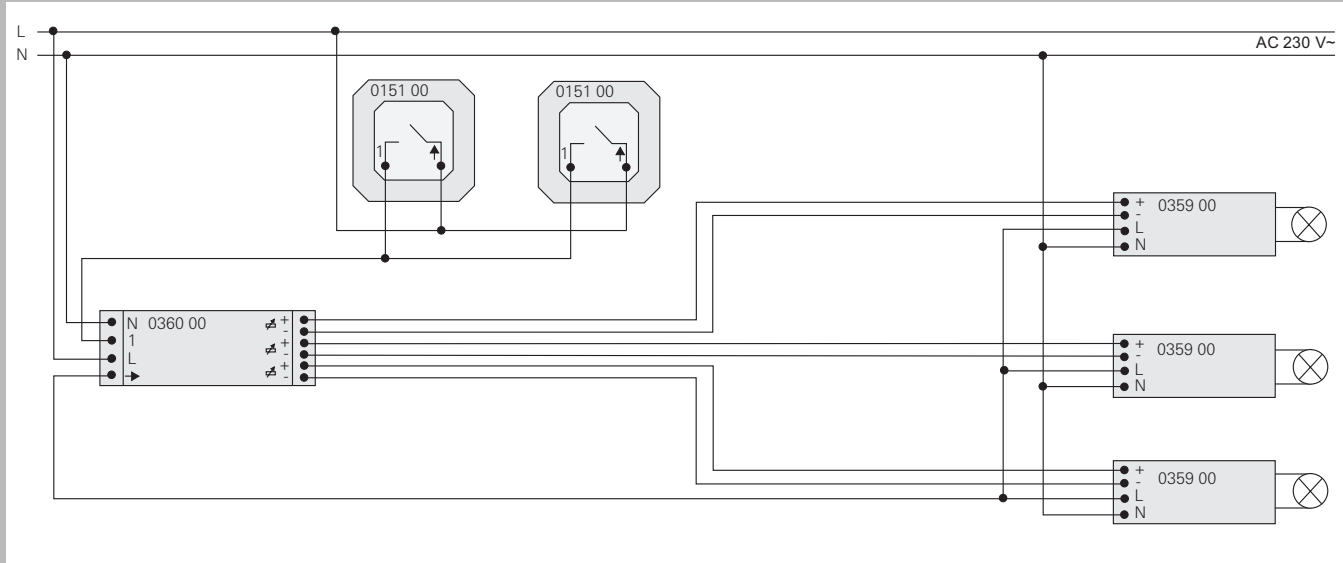
Встраиваемый модуль управления с выходом управления 1-10 В с электронным трансформатором со входом управления 1-10 В
