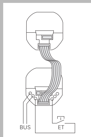
Подключение квартирной станции при соединении „Шлейф“
