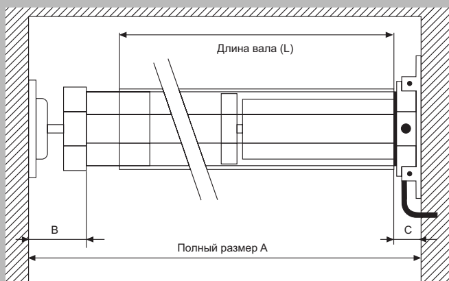
Длина вала L = A - (B + C)
