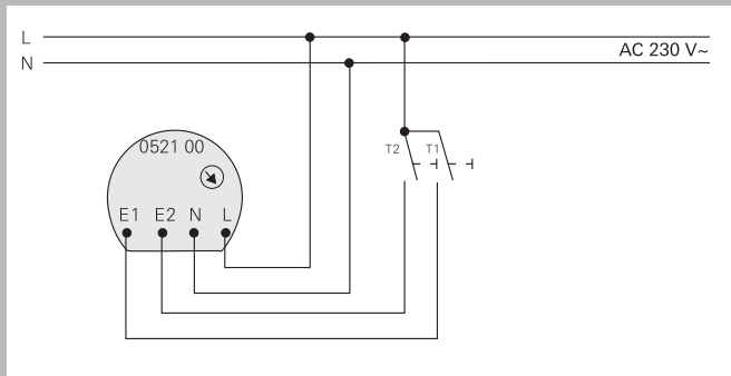
Подключение кнопочных выключателей (выключатель с нормально-разомкнутым контактом T1, T2)
