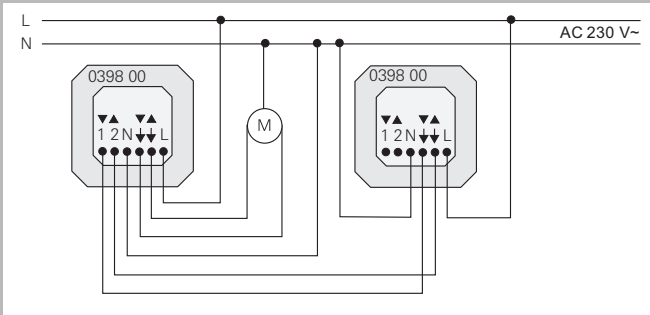
Подключение вставки управления жалюзи с дополнительным устройством
