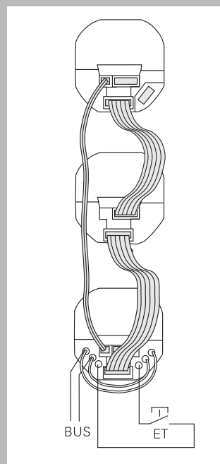
Подключение квартирной станции при соединении „Шлейф“
