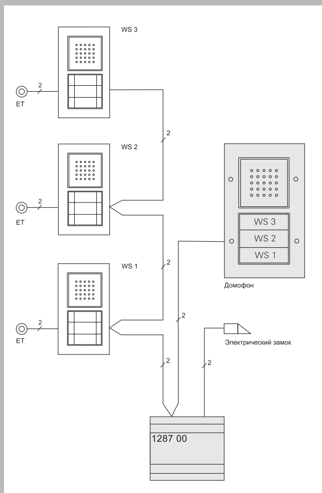
Способ соединения „Последовательная цепь“
