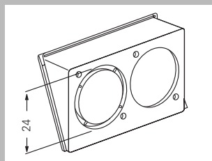
Вставка к парному круглому разъему XLR, серия "D", серия "Speakon" NL 4 MP (Neutrik) 0055 00
