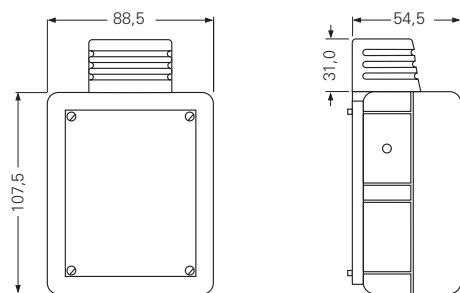
Ответительные коробки
