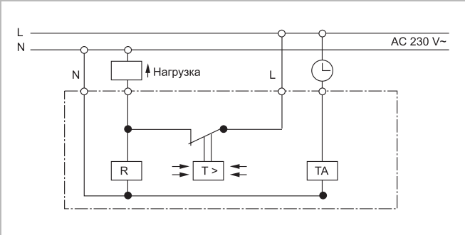
Термостат для помещений 230/10 (4) А~ с размыкающим контактом
