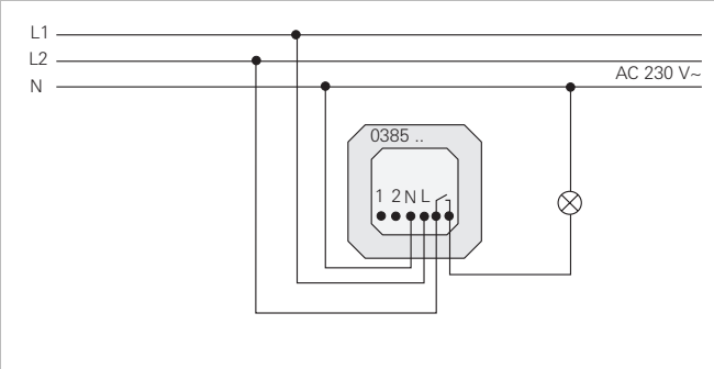
Подключение к 2 фазам. Вставка таймера оборудована беспотенциальными контактами.
