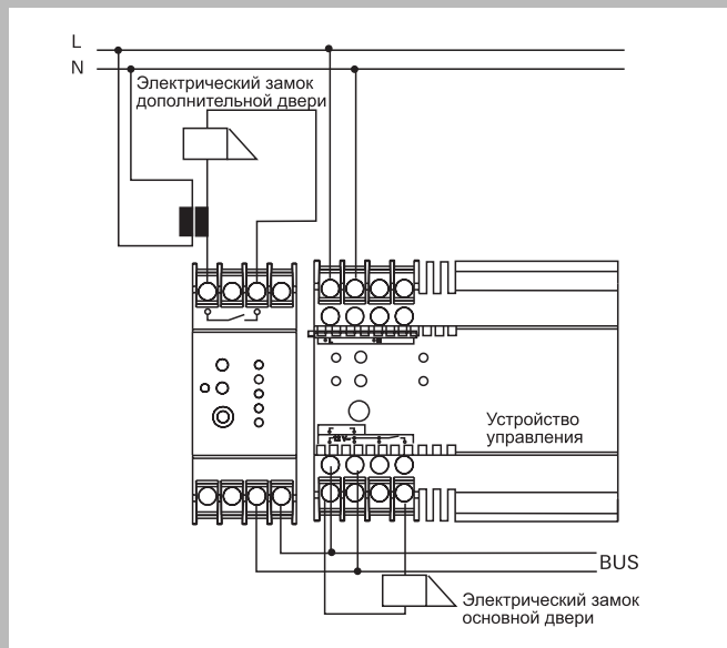
Соединение устройства открывания дверей с дополнительным реле
