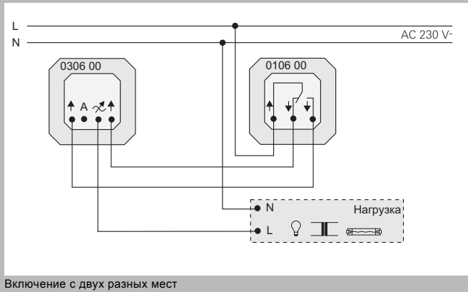
Включение с двух разных мест
