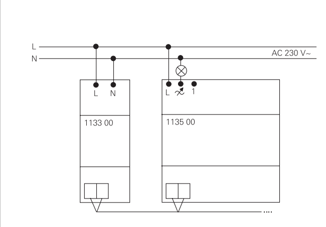
Подключение универсального светорегулятора REG с радиоуправлением
