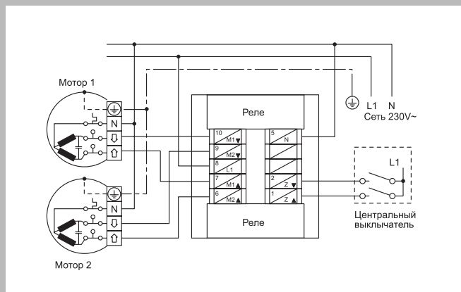
Схема соединения разделительного реле 0386 00
