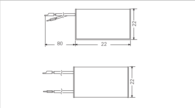
Модуль автомата защиты от перенапряжения 230 В~, 50 Гц
