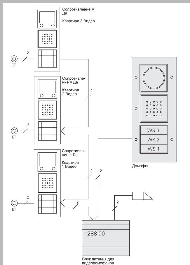
Соединение „Последовательная цепь“
