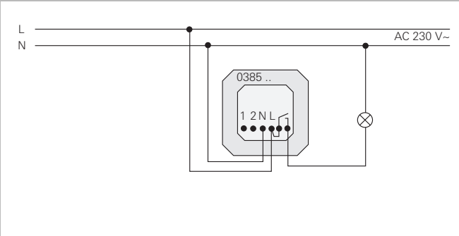
Фаза "L" соединяется с реле входа („перемычка")
