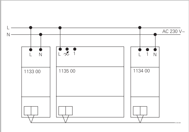
Подключение радиоприемного модуля REG
