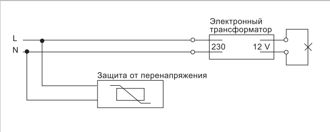
Режим переключения с защитой от перенапряжения
