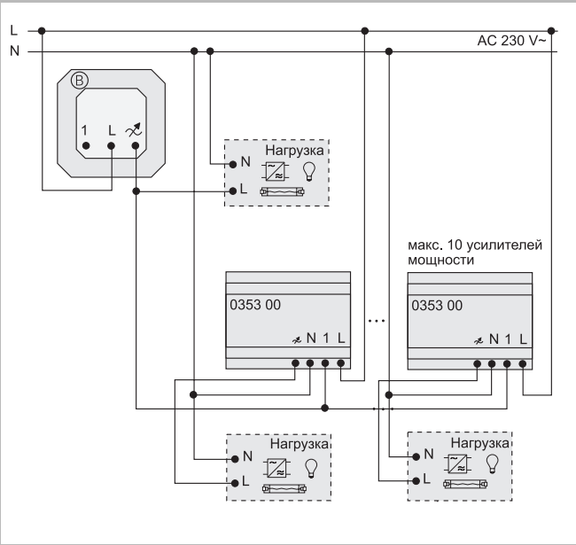
Параллельное включение нескольких усилителей мощности Tronic
