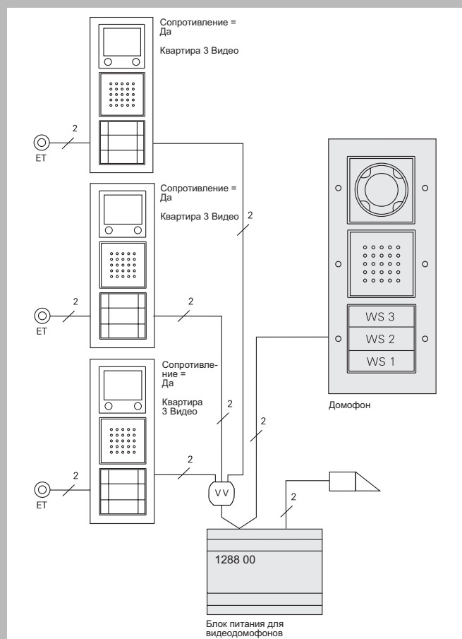
Соединение „Шлейф“
