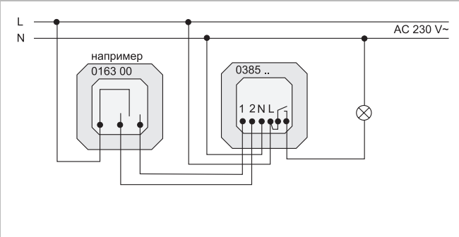
Подключение с механическим дополнительным устройством. Фаза "L" соединяется с реле входа („перемычка")
