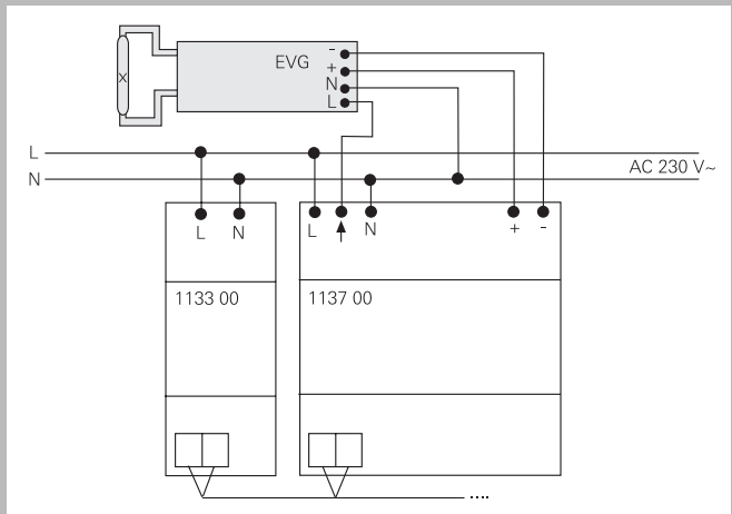
Подключение исполнительного радиоустройства 1-10 В REG
