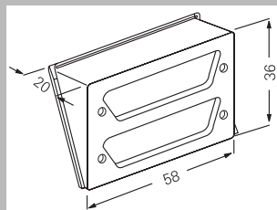
Вставка к D-Subminiatur 0050 00
