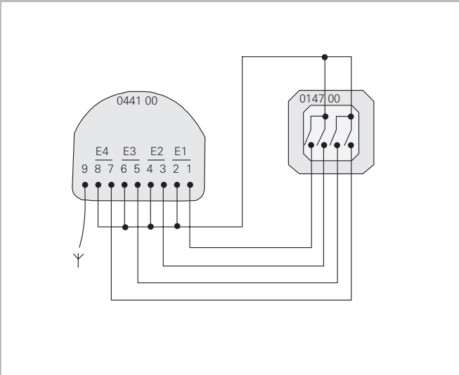
Соединение многофункционального радиопередатчика с 4-канальной вставкой кнопочного выключателя.
