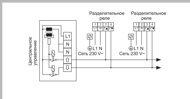
Параллельное включение разделит. реле 0861 00
