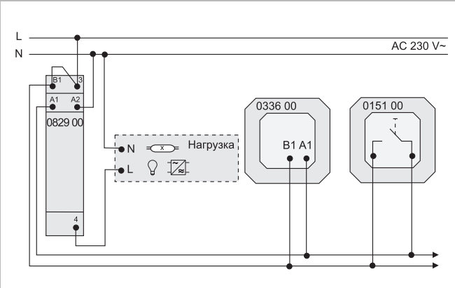
Подключение 4-проводного выключателя (переключаемая фаза)
