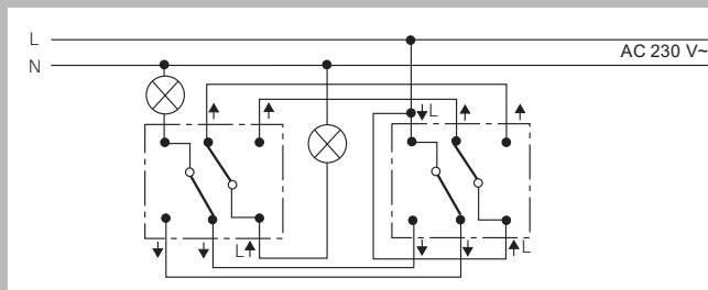
Переключатель с двух мест
