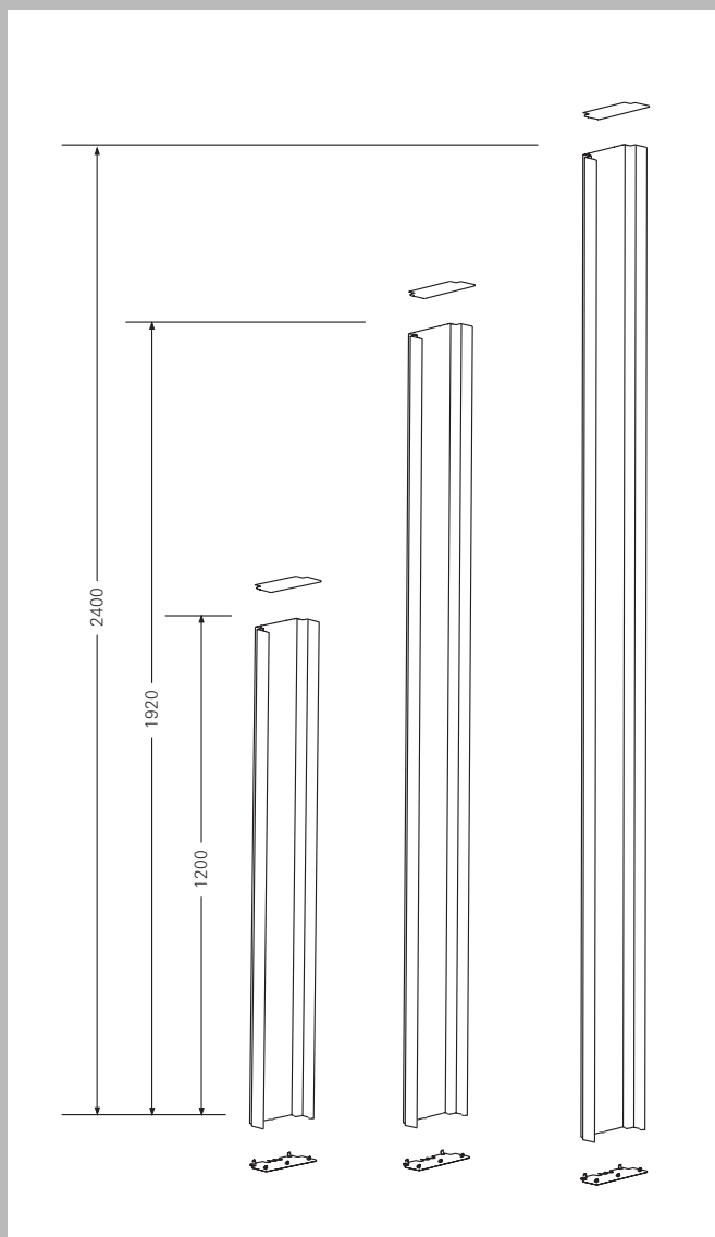
Монтажный профиль для установки 5, 8 и 10 модулей
