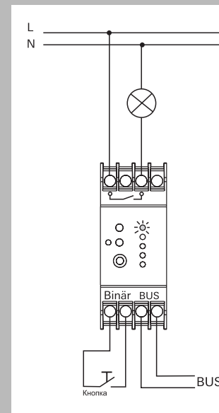
Подключение осветительного прибора
