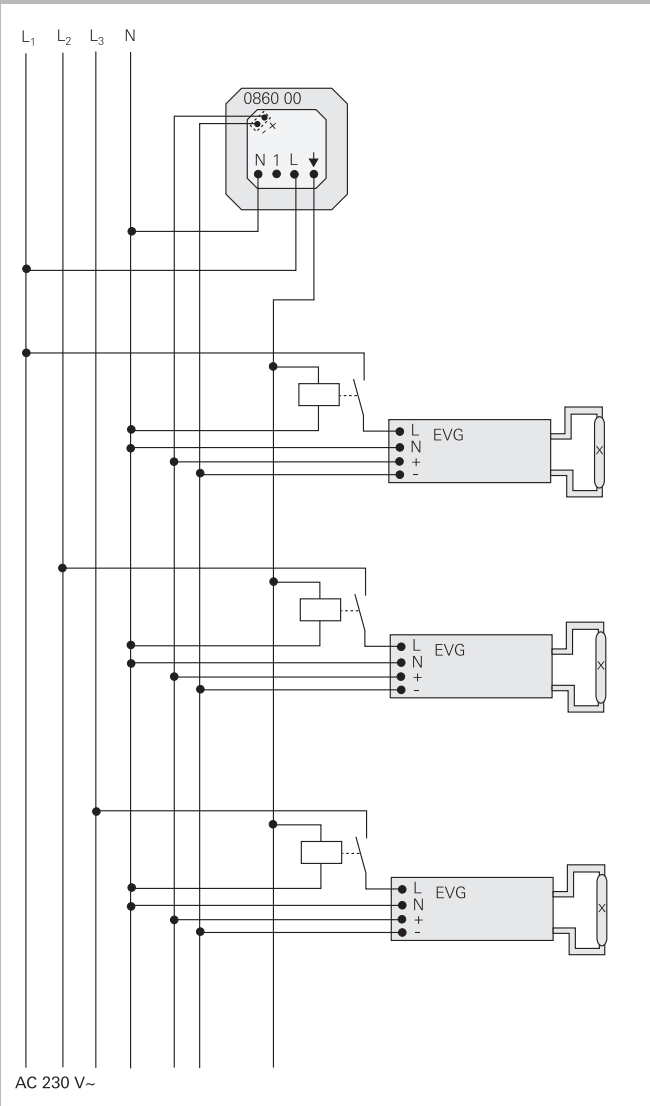
Распределение нагрузки в нескольких фазах. При многофазном соединении соблюдайте полярность.
