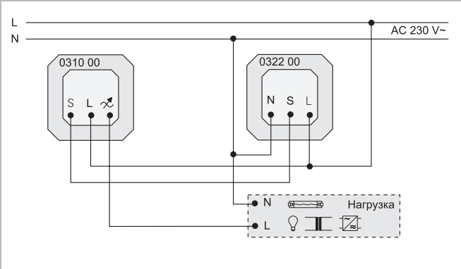
Соединение вставки дополнительного устройства к универсальному поворотному светорегулятору
