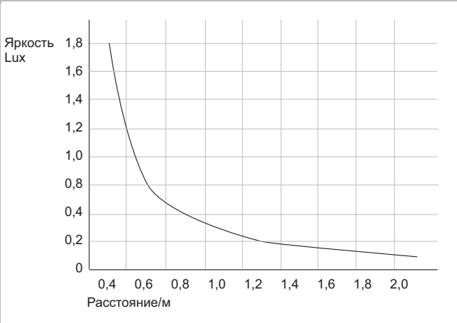
Зависимость яркости от расстояния до светильника по направлению луча
