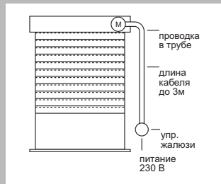
Подключение скатывающего устройства с шнуровым выключателем
