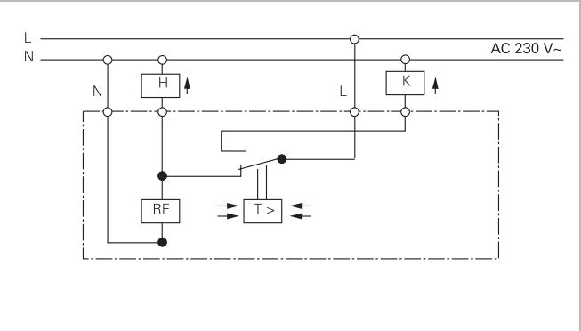
Термостат для помещений 230/5 (2) А~ с переключающим контактом
