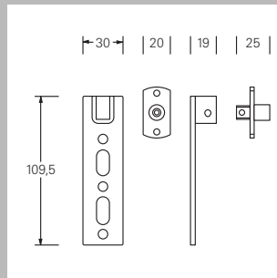
Габариты сборной опоры короба 0827 00
