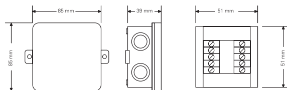
Габариты разделит. реле 0386 00, 0387 00
