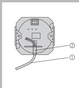
Сеть открытой электропроводки, вариант 2 (кнопочный выключатель управления с преобразователем сигналов датчиков)
