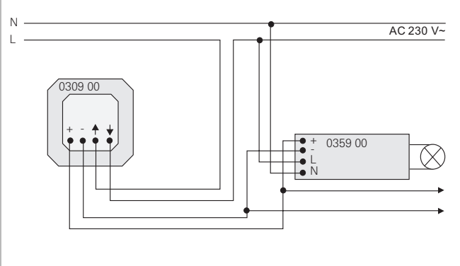
Электронный потенциометр 1-10 В с электронным трансформатором с встроенным входом управления 1-10 В
