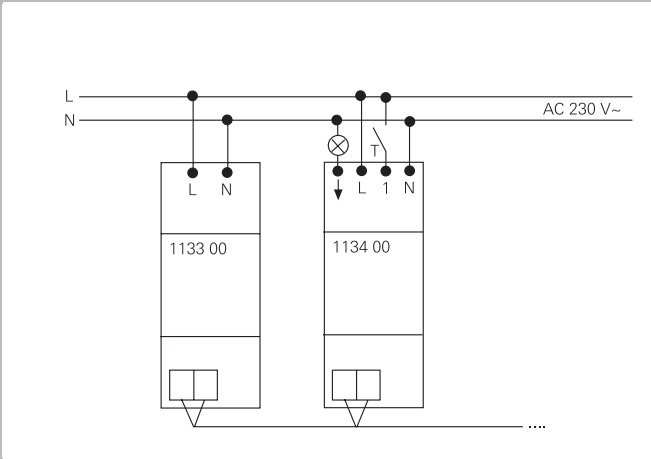
Подключение радиокоммутатора 1-канального REG
