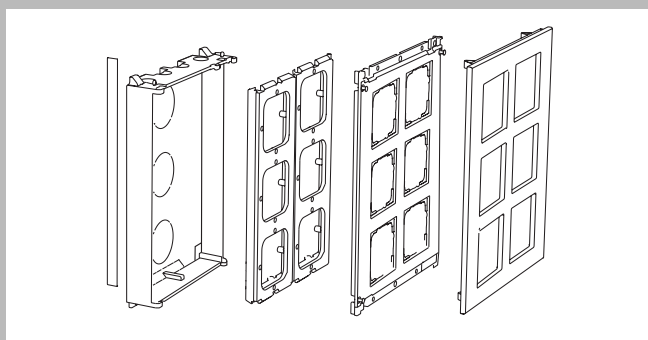
Унифицированный модуль для установки шести вставок для скрытой электропроводки серии System 55 в модульные функциональные стойки.
