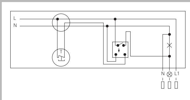
Параллельное включение с автоматическим выключателем лестничного освещения или импульсным выключателем Освещение включается или автоматическим выключателем лестничного освещения или сторожевым устройством.
