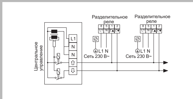
Параллельное включение разделительного реле 0387 00
