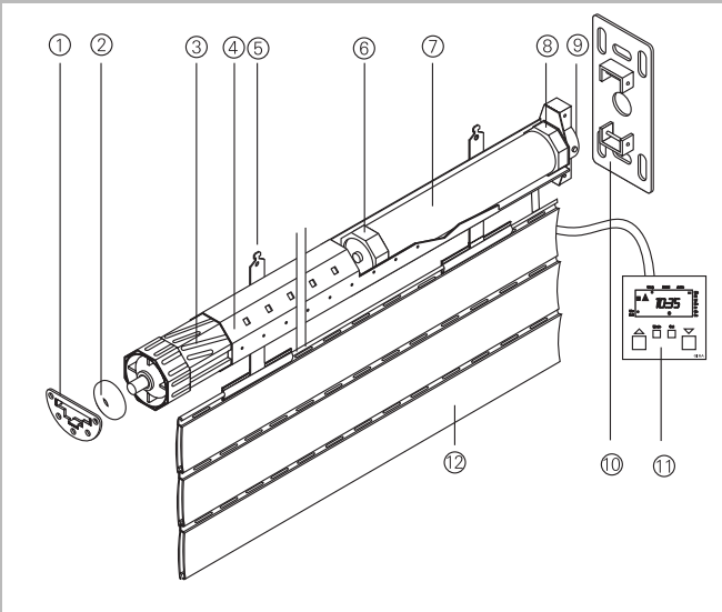
Схема установки коакс. мотора
