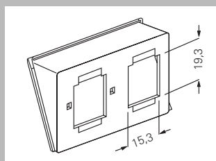
Вставка к модульному разъему Jack/Western Technik, AMP/Radiall, 2-секционн. 0053 00
