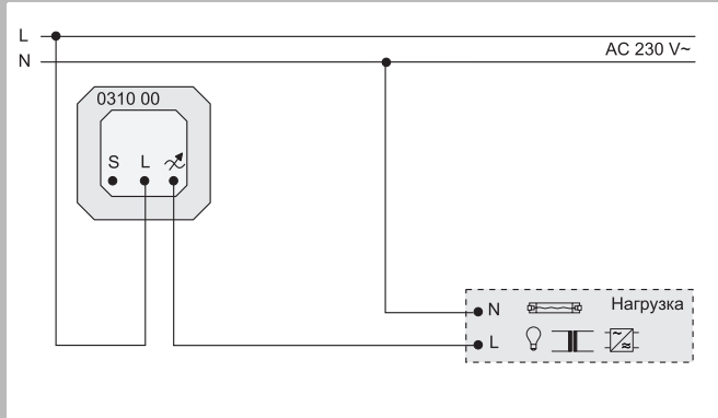
Подключение универсального поворотного светорегулятора
