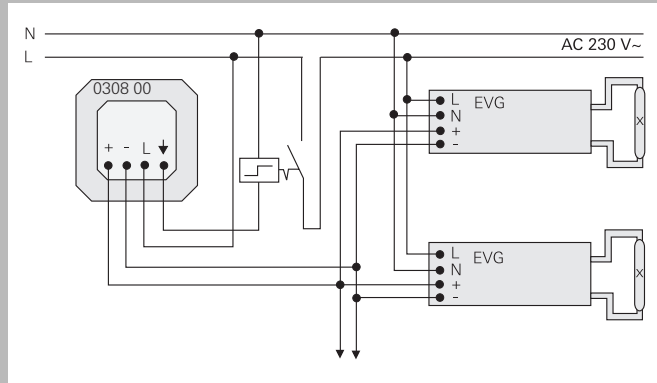
Подключение электронного потенциометра с функцией кнопочного выключателя на EVG
