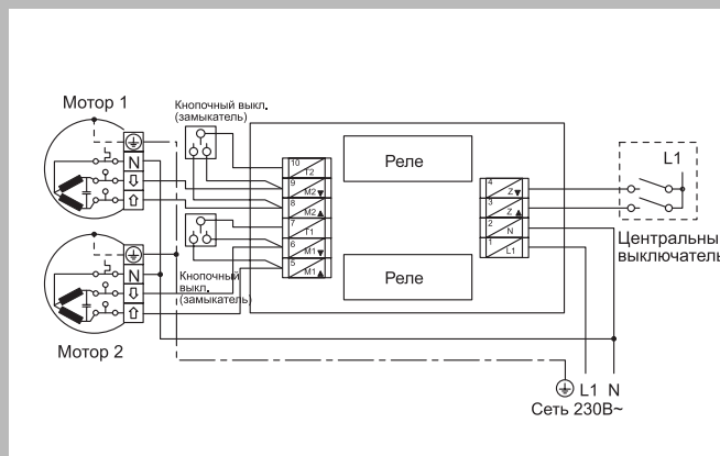
Схема соединения разделительного реле 0861 00
