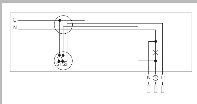
Автоматическое или ручное управление с помощью двухклавишного выключателя
