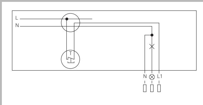
Подключение сторожевого устройства и включаемых системой потребителей мощности
