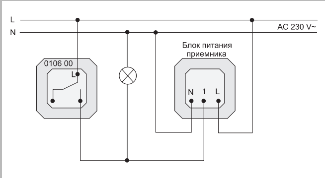
Выключатель на параллельном входе 230 В блока питания приемника
