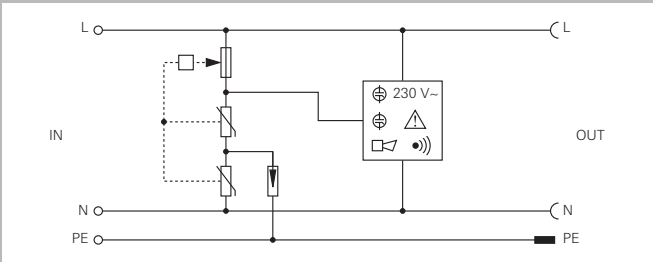
Электрическая схема
