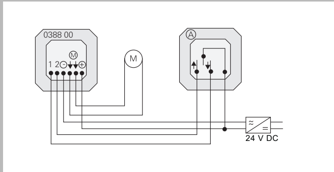
Подключение вставки управления жалюзи 24 В пост. тока с механическим дополнительным устройством (кнопочный выключатель жалюзи с механической сцепкой).
