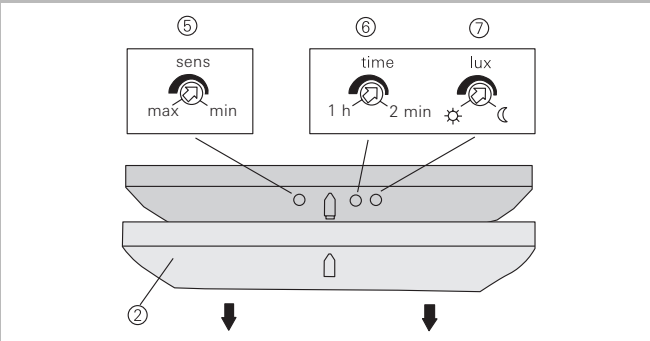
Расположение регуляторов
