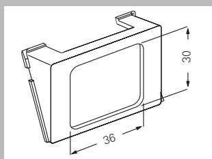
Вставка к AMP/ACO Communications Outlet) Подходит только к разъемам, направленным под углом 30°. 0059 00
