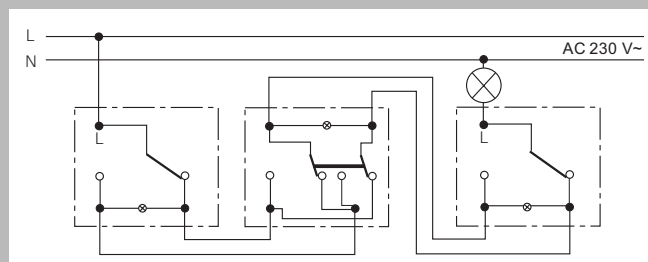
Перекрестный выключатель
